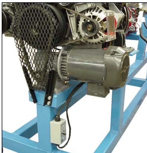
MOTEUR ÉLECTRIQUE
